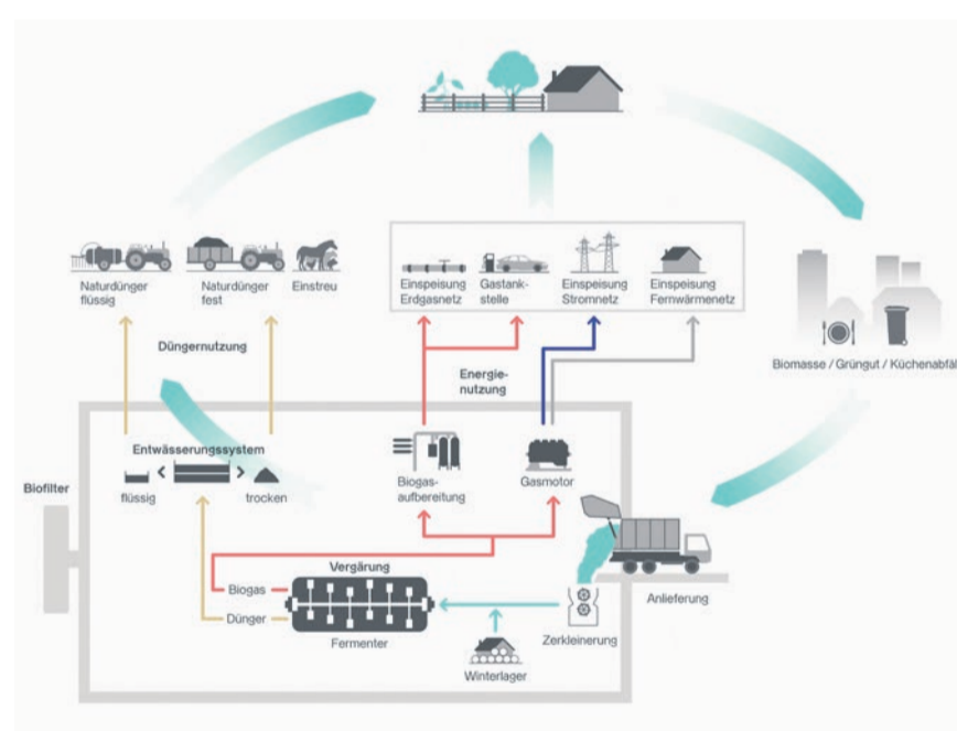
Der Kreislauf einer Vergärungsanlage.
